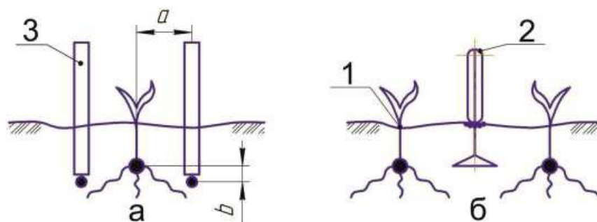
Рис. 2. Схемы внесения удобрений: вблизи рядка (а) и посередине междурядий (б): 1 – рядок растений; 2 – долотообразная лапа; 3 – подкормочный нож; а – расстояние от рядка до подкормочного ножа; б – глубина заделки удобрений
