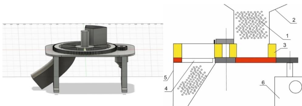
Рис. 3D модель и конструктивно-технологическая схема экспериментального дозатора:
