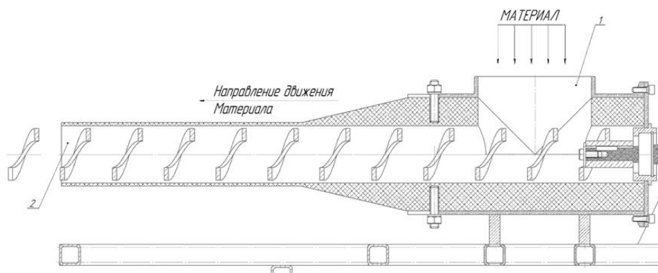
Рис. 3. Принцип действия лабораторного спирально-винтового дозатора
