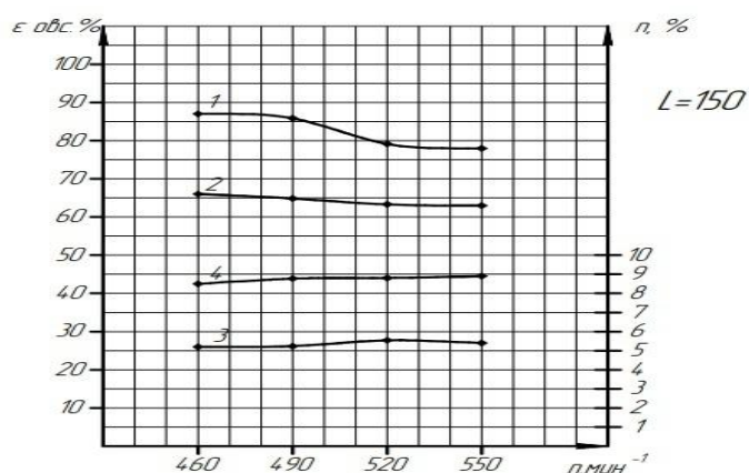
Рис. 3. Закономерности изменения степени отделения семян овсяга из основной фракции-1, выхода основной-2 и промежуточной-3 фракций и потерь семян в отходы -4 при длине направителя 150 мм
