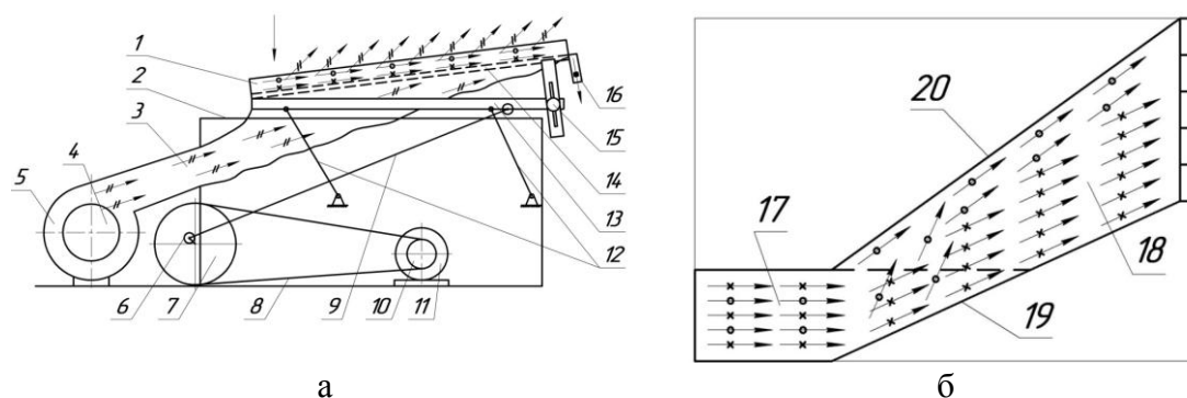
Рис. 1. Экспериментальный пневмосортировальный стол: а) – устройство: 1 – дека; 2 – рама; 3 – воздуховод; 4 – заслонка; 5 – вентилятор; 6 – эксцентрик; 7, 10 – шкив; 8 – ремень; 9 – шатун; 11 – электродвигатель; 12 – подвеска; 13 – рамка; 14 – воздуховывравнивающая поверхность; 15 – механизм регулирования продольного угла наклона деки; 16 – приемники фракций; б) – технологическая схема деки, вид сверху: 17 – зона предварительного расслоения; 18 – зона транспортирования; 19,20 – стенки деки
