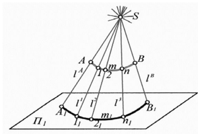
Рис. 3. Аксонометрическое изображение конической поверхности: S – вершина; m – направляющая кривая линия; l – образующая – прямая линия
