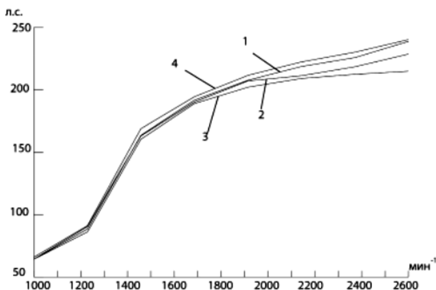
Рис. 2. Изменение эффективной мощности от частоты вращения: 1 – АМОВТ с минимальным износом; 2 – АМОВТ со средним износом; 3 – АМОВТ с максимальным износом; 4 – эталонная АМОВТ
