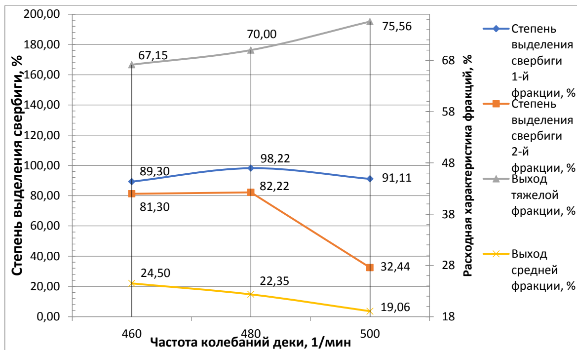
Рис. 1. Закономерности изменения степеней выделения примесей из фракций пшеницы и их выходы при отделении семян овсюга (а) и свербиги (б)
