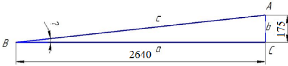
Рис. 4. Угол продольного крена кузова автомобиля Volvo C30
