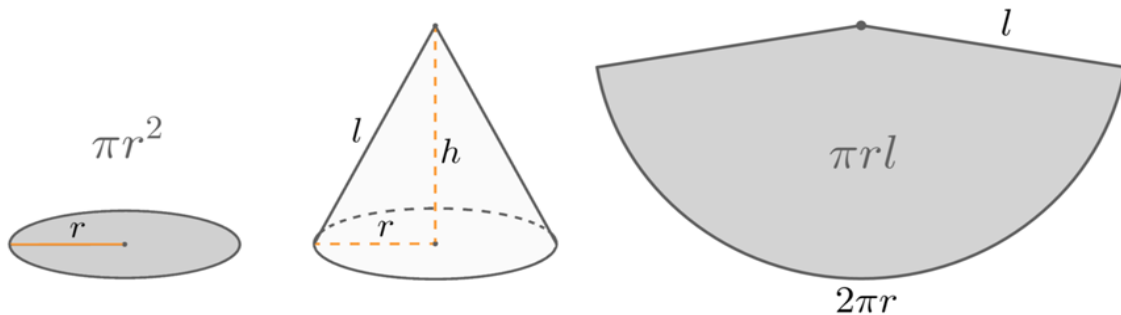
Рис. 2. Развертка конуса
