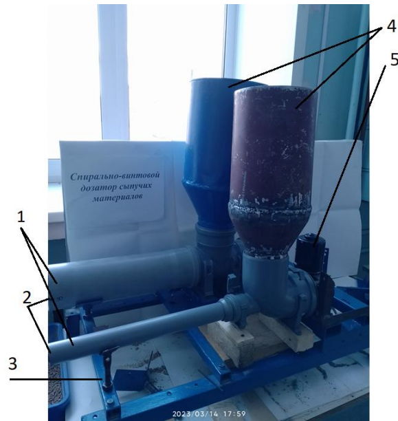
Рис. 2. Общий вид экспериментальной лабораторной установки: 1 – цилиндрический корпус, 2 – спираль, 3 – рама, 4 – бункер с загрузочной горловиной, 5 – моторредуктор 16.3730, 7
