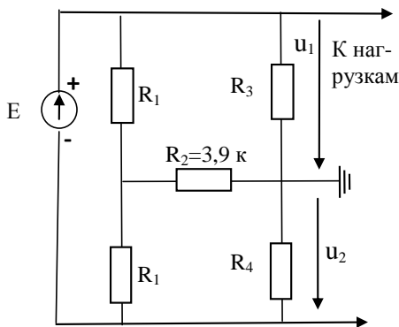
Рисунок 1 – Классическая схема контроля изоляции (УКИ)
