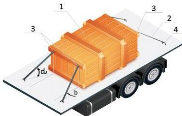
Рис. 3. Крепление груза прямой увязкой: 1 – груз; 2 – средство крепления; 3 – увязочное устройство на грузе; 4 – точка крепления на платформе
