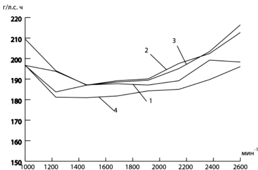
Рис. 3. Изменение удельного расхода топлива от частоты вращения: 1 – АМОВТ с минимальным износом; 2 – АМОВТ со средним износом; 3 – АМОВТ с максимальным износом; 4 – эталонная АМОВТ
