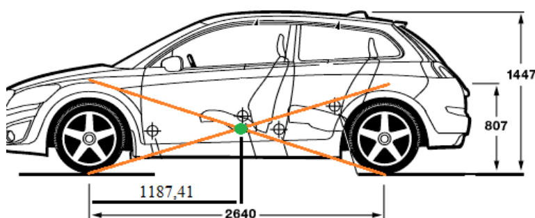
Рис. 3. Ось крена автомобиля Volvo C30
