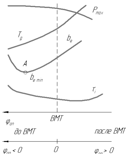
Рис. 1. Регулировочная характеристика дизельного двигателя по углу опережения впрыска топлива: P_{max} – максимальное давление сгорания; T_g – температура отработавших газов; b_e – удельный расход топлива; \tau_i – период задержки самовоспламенения
