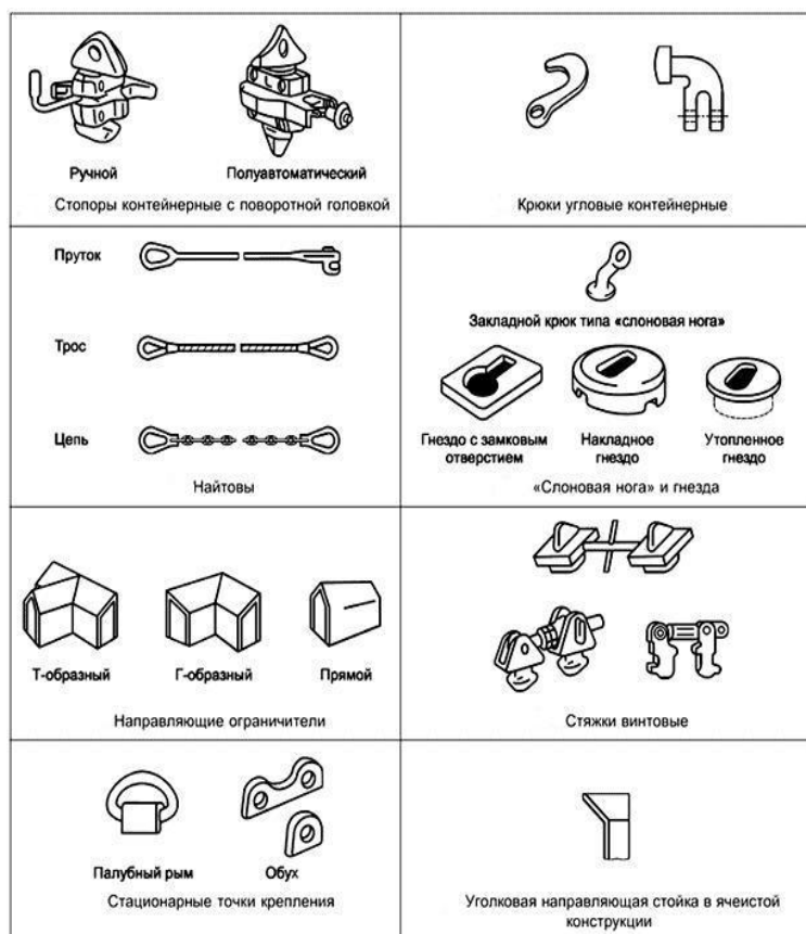
Рис. Примеры типовых устройств для крепления контейнеров
