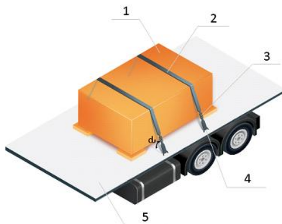
Рис. 2. Крепление груза с помощью прижимных ремней (способ увязки поверху): 1 – груз; 2 – прижимной ремень; 3 – натяжное устройство; 4 – точка крепления; 5 – платформа
