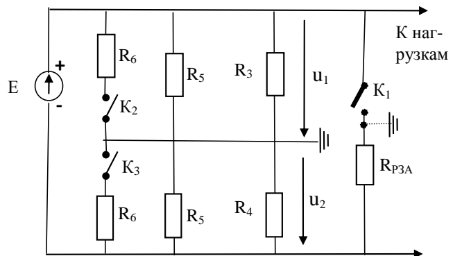
Рисунок 2 – Принципиальная схема устройства контроля изоляции с дополнительными сопротивлениями R_6
