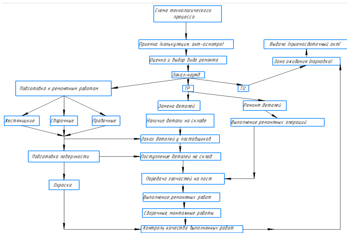
Рис. 2. Схема технологического процесса
