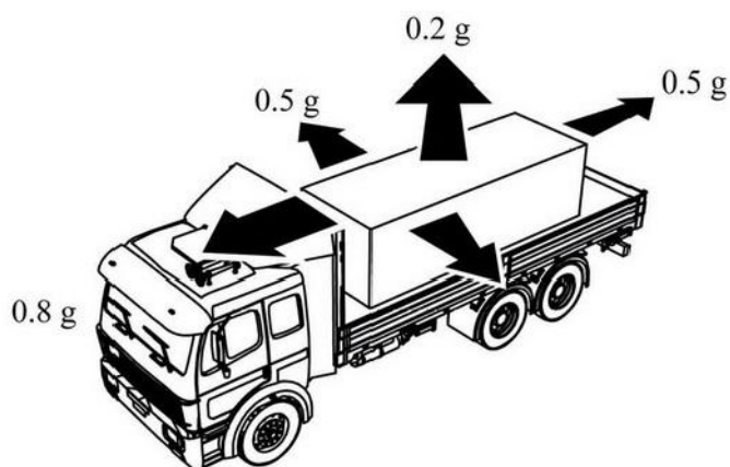
Рис. 1. Максимальные инерционные силы, действующие на груз
