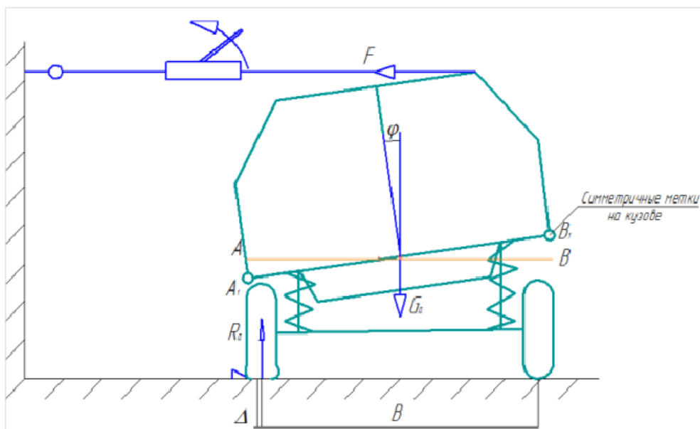
Рис. Метод опрокидывания на платформе
