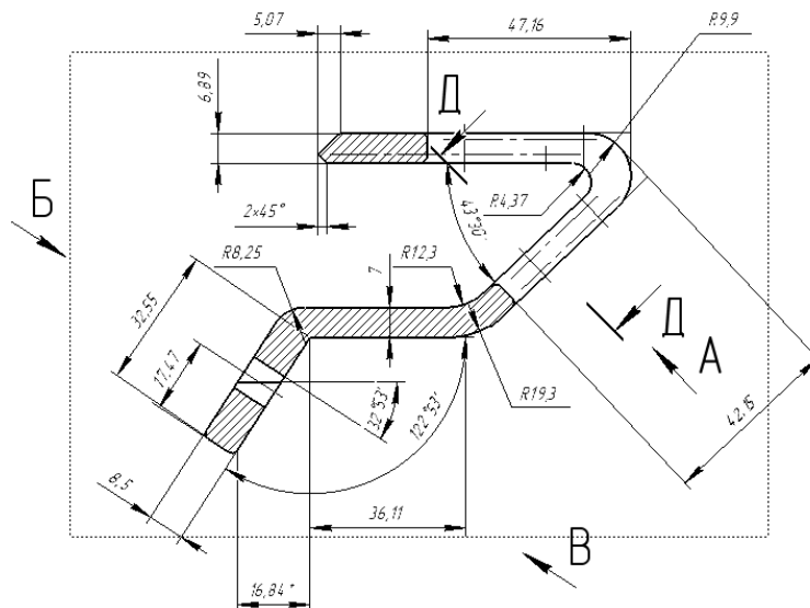
Рис. 3. Чертёж детали в nanoCAD
