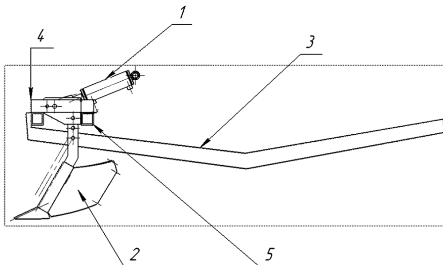
Рис. 2. Схема устройства для возврата картофеля в гребни: 1 – гидроцилиндры, 2 – окучники, 3 – балки для крепления к трактору, 4 – крепежи гидроцилиндров, 5 – каркас
