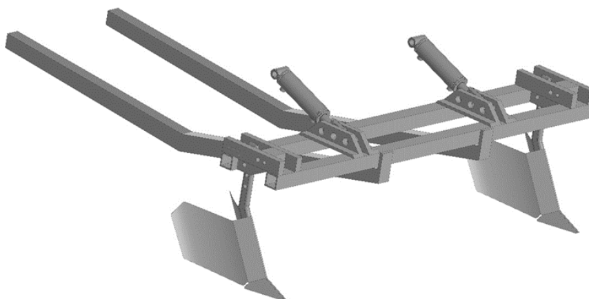
Рис. 3. 3D модель устройства для возврата картофеля в гребни
