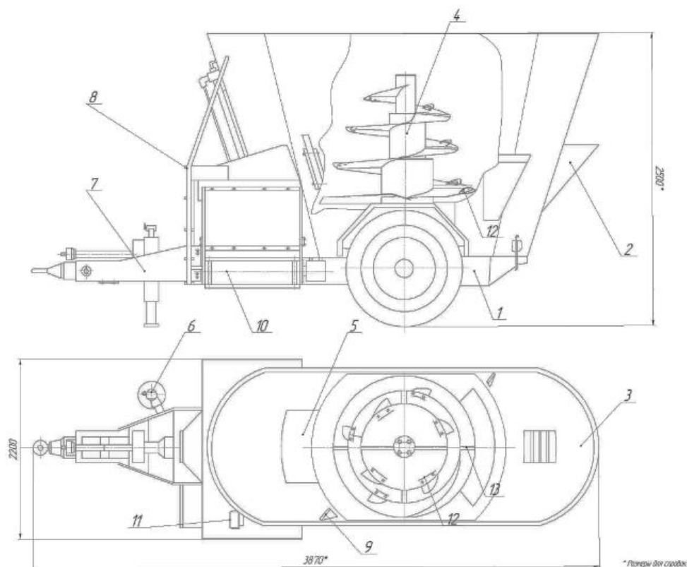
Рис. 1. СРК–11В с дополнительными ножами и пластинами
