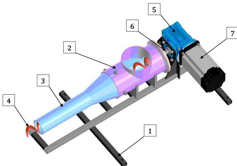
Рис. 2. Лабораторный спирально-винтовой дозатор минеральных удобрений
