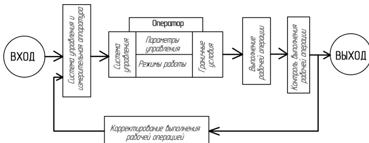
Рис. 1. Блок схема ручного управления строительной машиной
