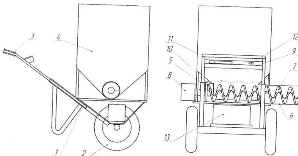
Рис. 7. Раздатчик концкормов со спирально-винтовым дозатором:
