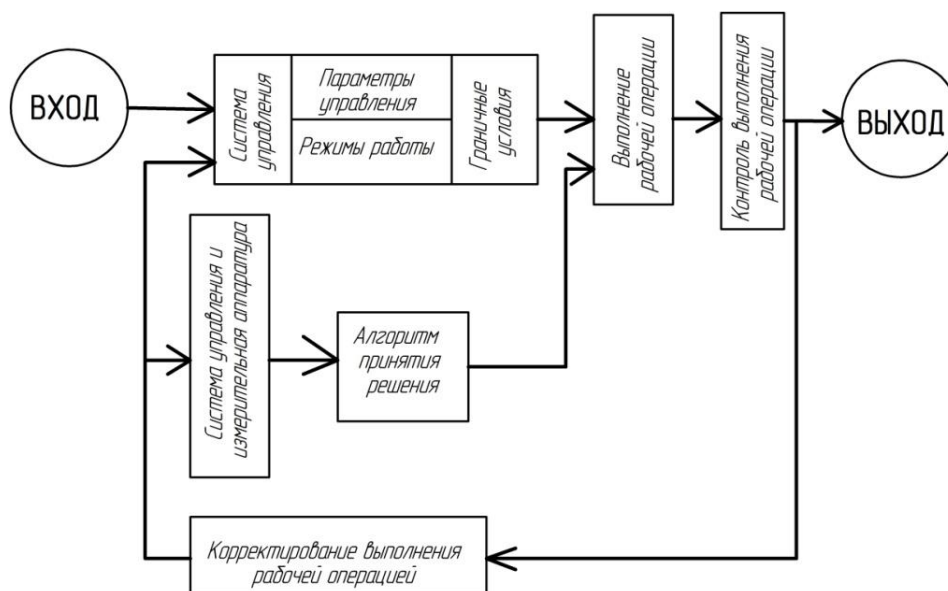
Рис. 2. Блок схема автоматической системы управления строительной машины
