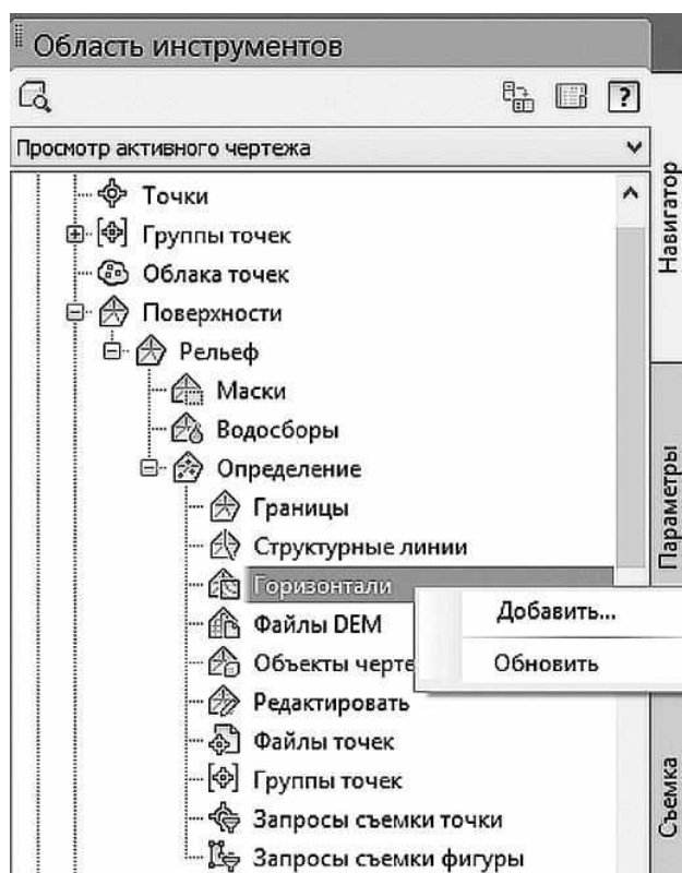
Рис. 1.21. Определение поверхности при помощи исходных горизонталей
