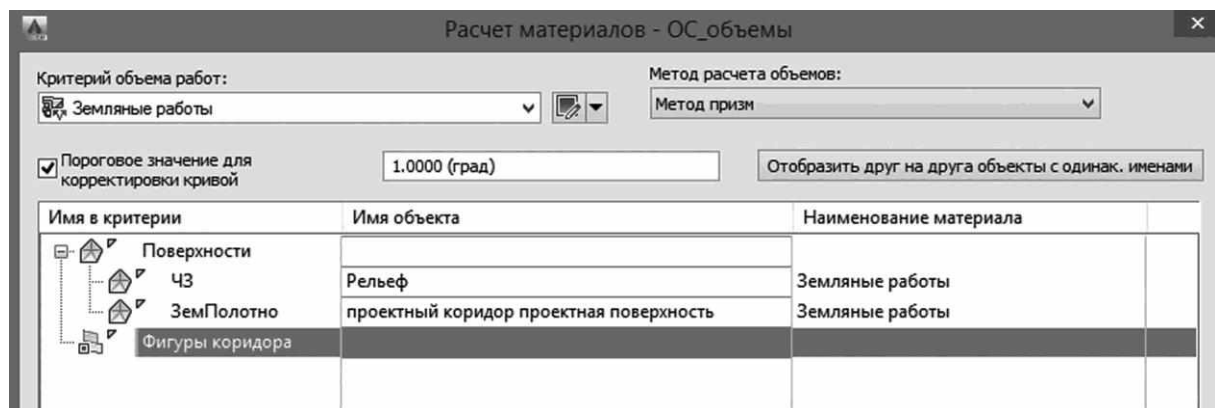
Рис. 5.7. Окно параметров для расчета материалов
