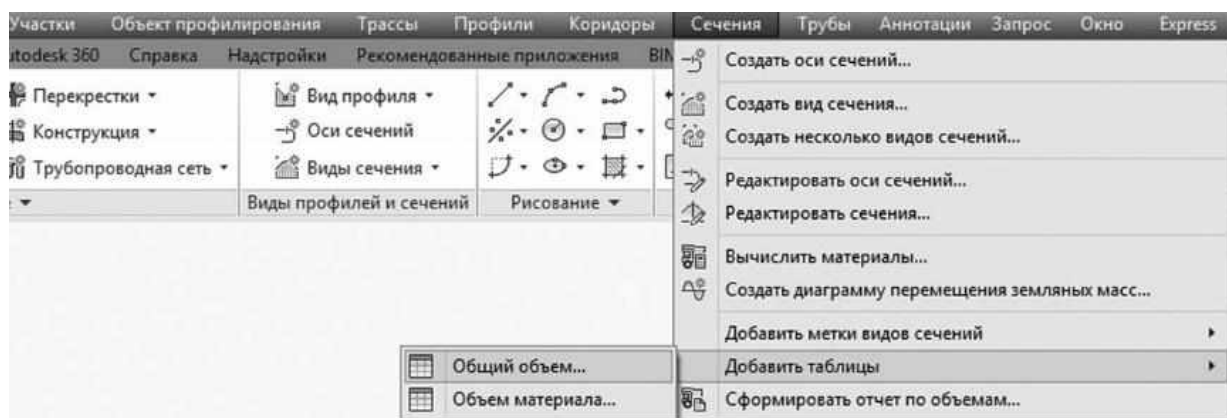
Рис. 5.9. Меню параметров оси сечений для добавления таблицы объемов
