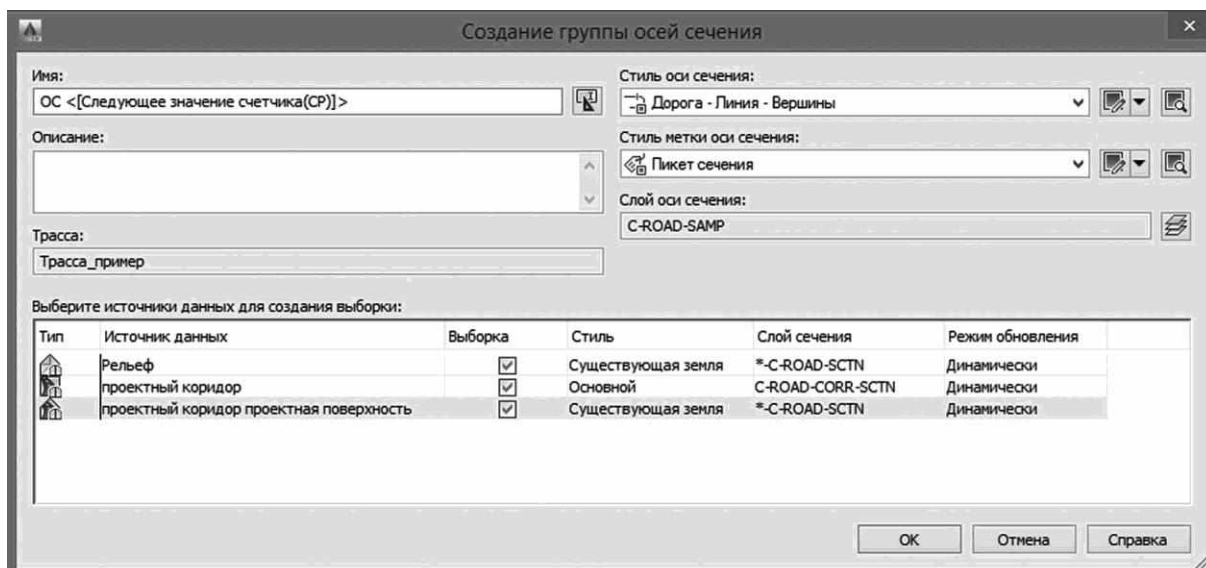
Рис. 5.2. Окно создания группы сечений
