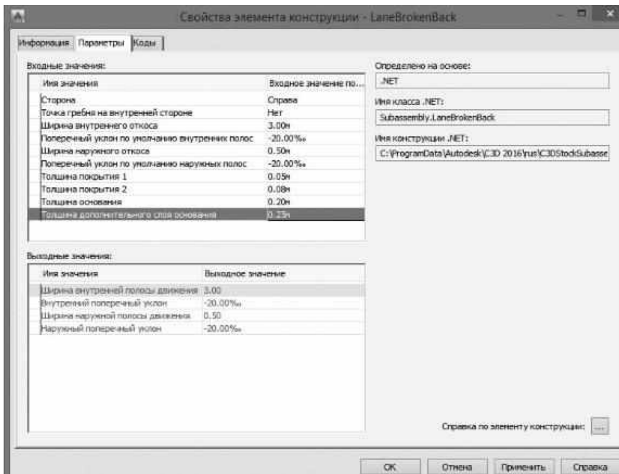
Рис. 4.5. Окно свойств элемента конструкции
