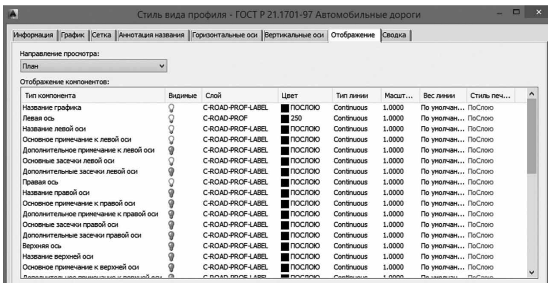
Рис. 3.3. Редактирование стиля вида профиля
