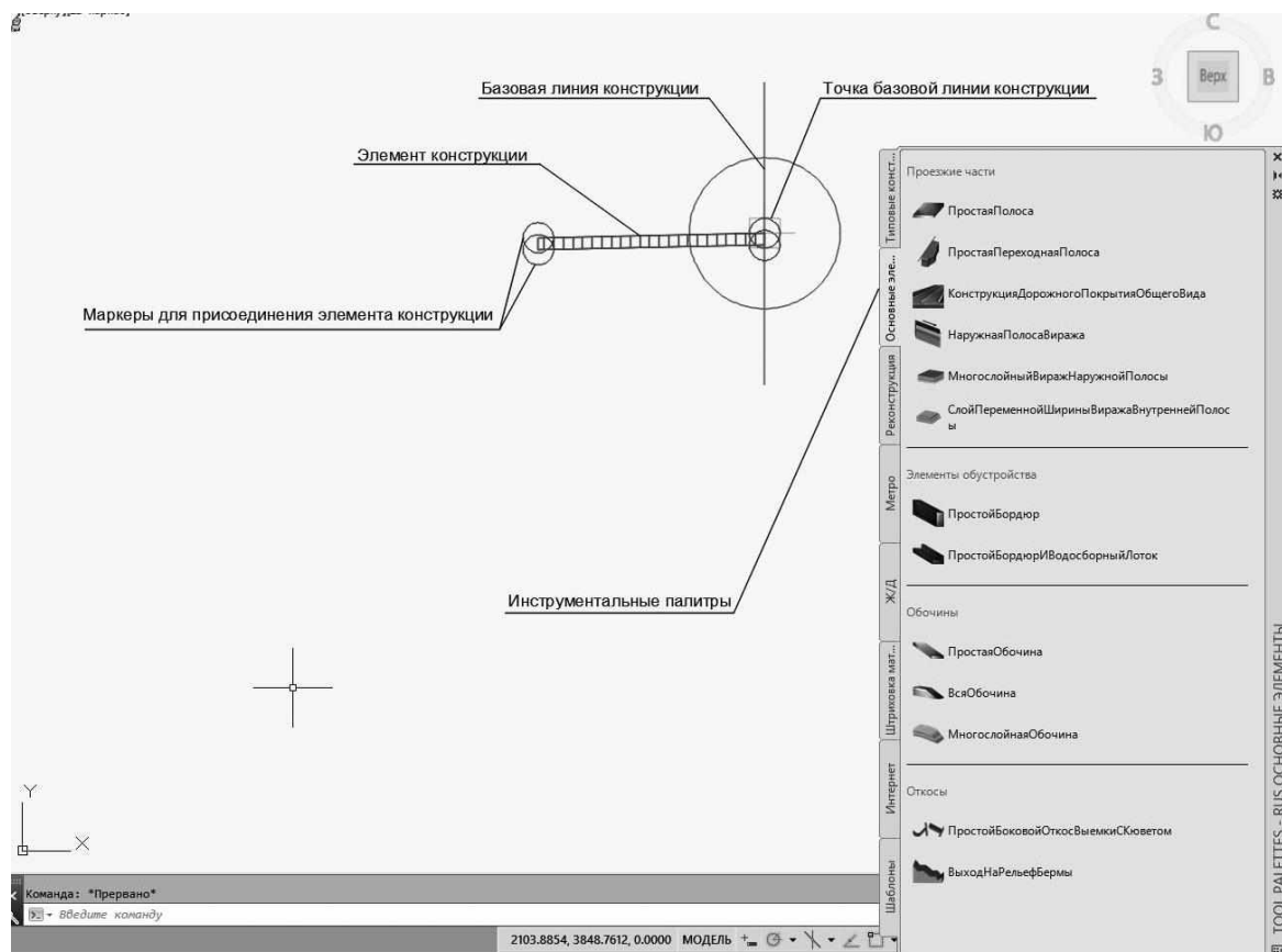
Рис. 4.1. Элементы конструкции поперечного профиля
