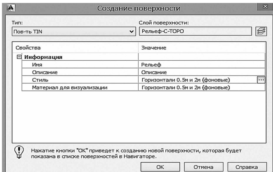
Рис. 1.13. Отображение свойств поверхности
