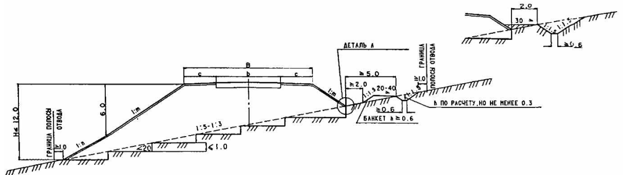
Рис. 4.1. Типовые поперечные профили земляного полотна
