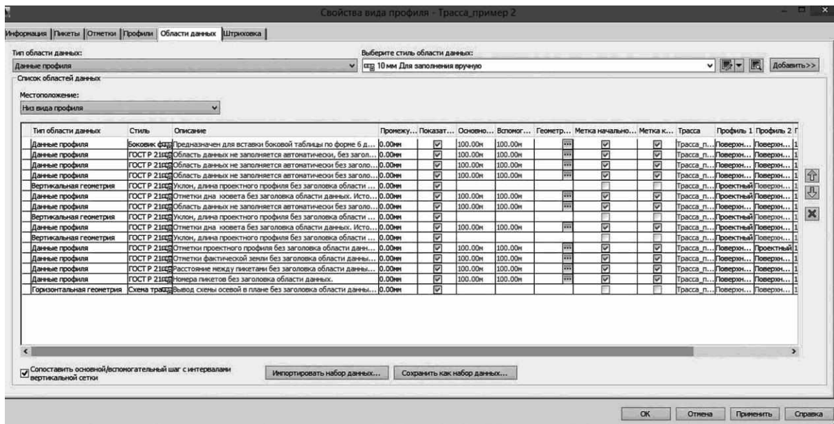
Рис. 3.12. Назначение данных вида профиля
