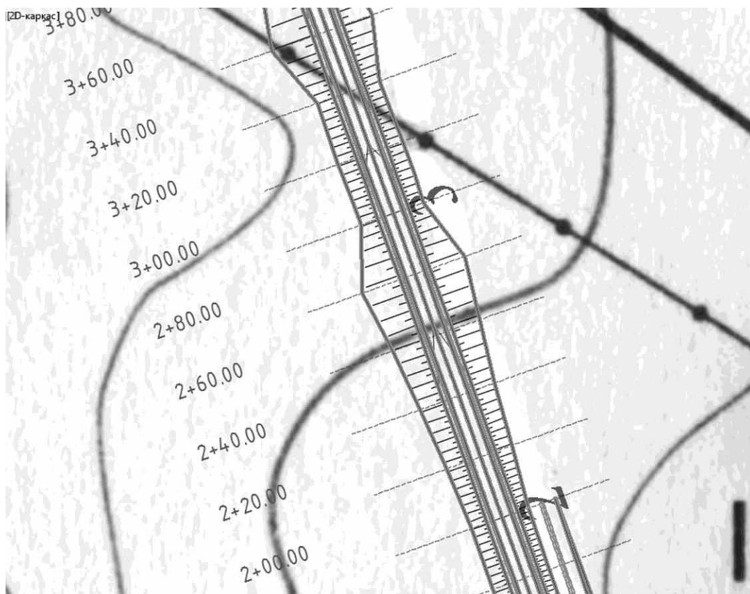
Рис. 5.5. Отображение сечений на чертеже
