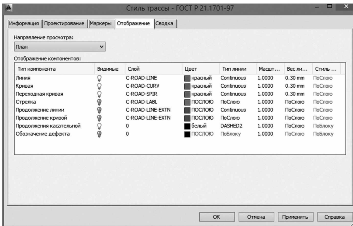
Рис. 2.6. Стили отображения трассы
