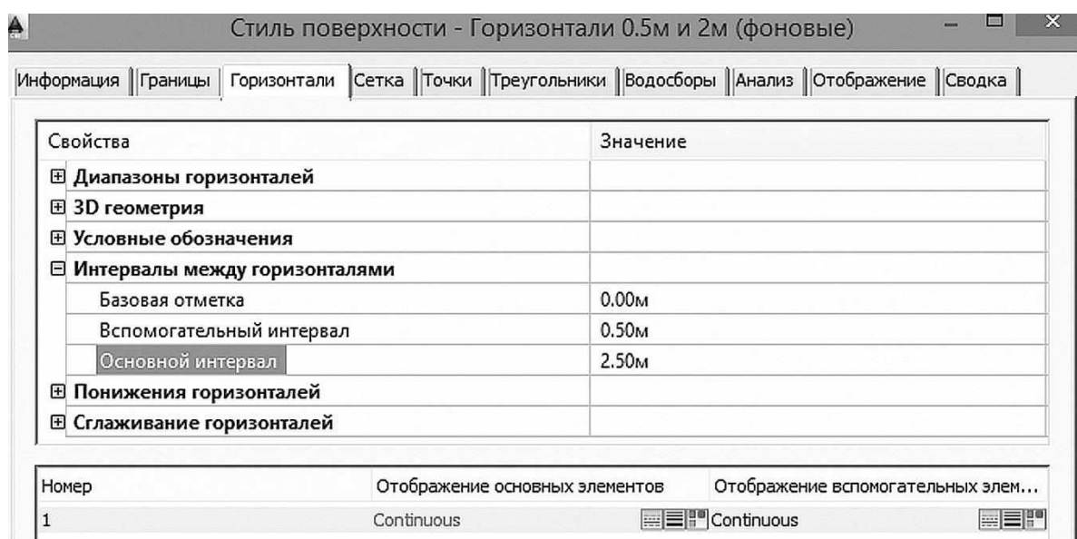
Рис. 1.23. Назначение интервала между горизонталями
