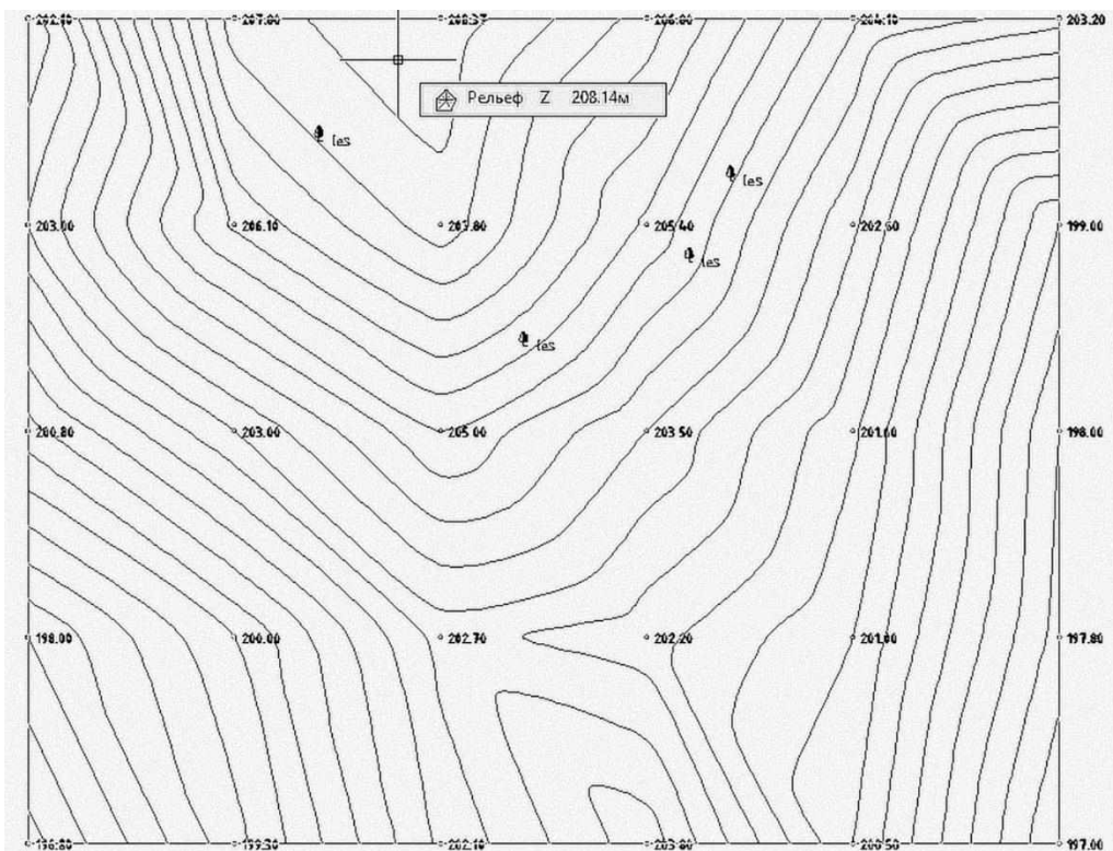
Рис. 1.15. Итоговая цифровая модель поверхности
