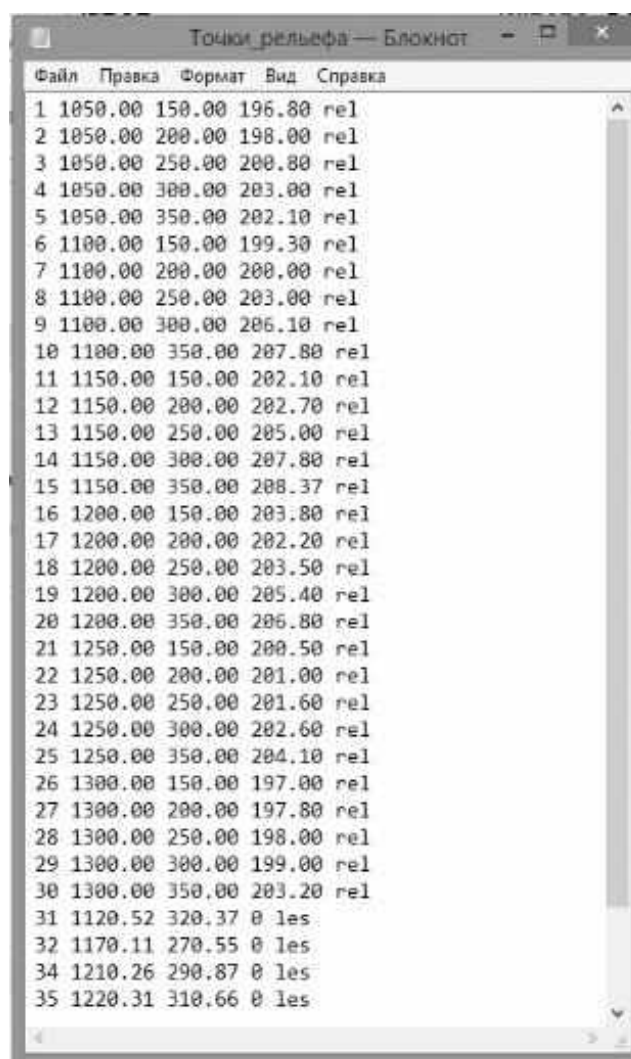
Рис. 1.2. Файл исходных точек рельефа
