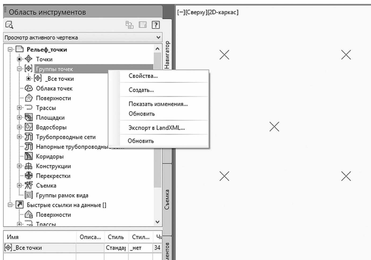
Рис. 1.7. Свойства групп точек
