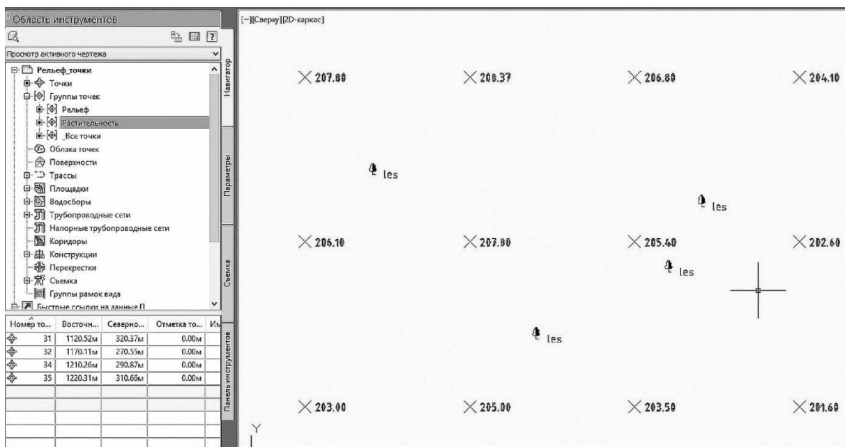
Рис. 1.11. Отображение точек ситуации на чертеже
