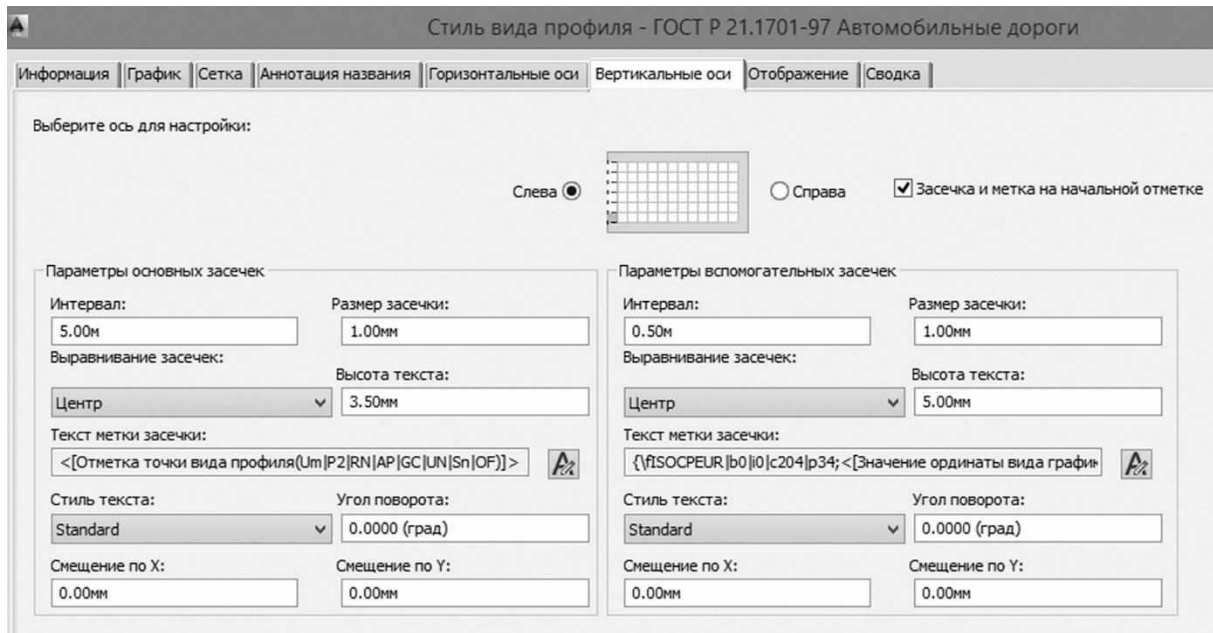
Рис. 3.4. Редактирование вертикальной оси сетки продольного профиля
