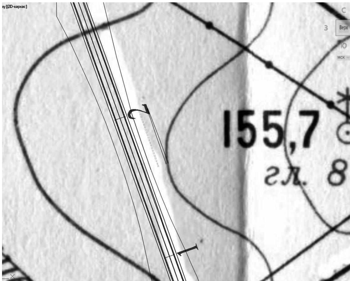
Рис. 4.11. Характерные линии коридора на плане трассы
