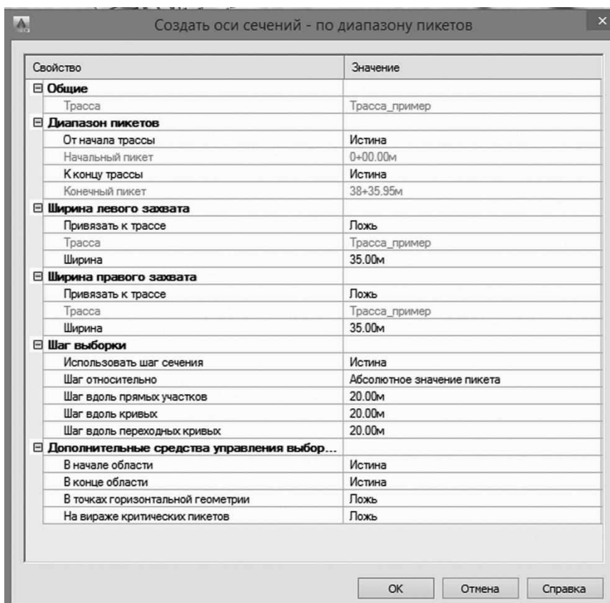
Рис. 5.4. Окно свойств оси сечений
