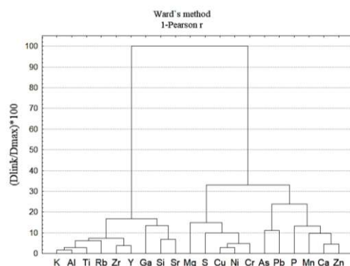
Рисунок 1. Дендрограмма кластерного анализа взаимосвязи химических элементов, нормированных по железу, в почвах и наилках пойм малых рек г. Перми (n = 80)
